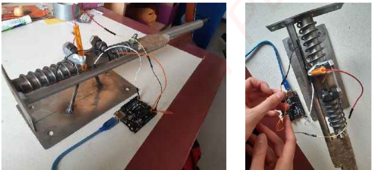
Figure 30 - Photographies de l'assemblage des ressorts avec le potentiomètre low-tech
