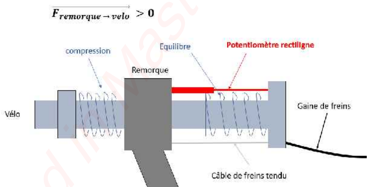
Figure 13 - Potentiomètre lors du freinage (2 ème modèle)
