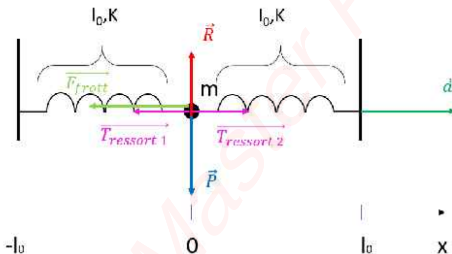
Figure 17 - Modélisation du système de ressort avec les forces exercées sur la remorque (2 ème modèle)
