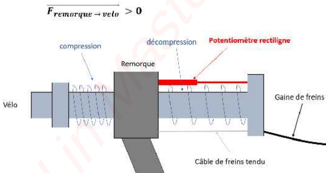
Figure 7 - Potentiomètre lors du freinage (1 er modèle)
