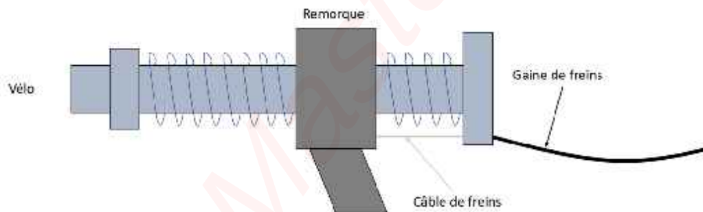
Figure 9 - Schéma de la remorque à l'équilibre (1 er modèle)
