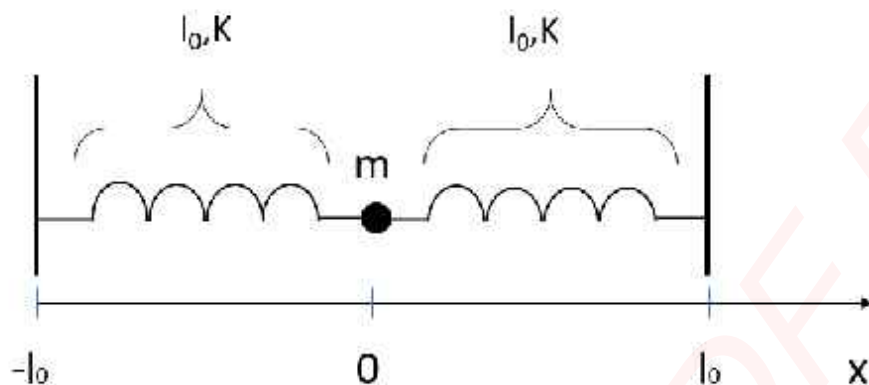
Figure 16 - Modélisation du système de ressort (2 ème modèle)
