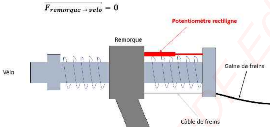
Figure 6 - Potentiomètre à l'équilibre (1 er modèle)
