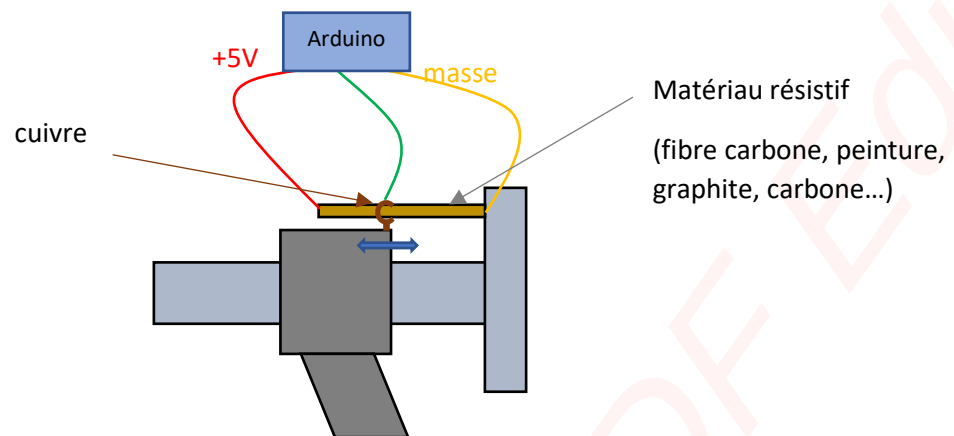
Figure 23 - Schéma du potentiomètre low-tech adapté à la remorque
