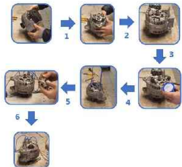
Figure 31 - Etapes de transformation d'un alternateur en moteur
