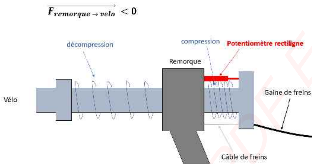
Figure 8 - Potentiomètre lors de l'accélération (1 er modèle)
