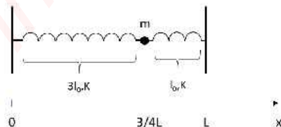
Figure 10 - Modélisation du système de ressorts (1 er modèle)
