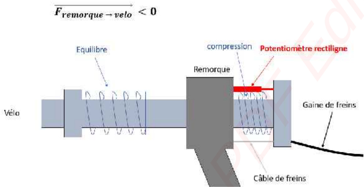
Figure 14 - Potentiomètre lors de l'accélération (2 ème modèle)
