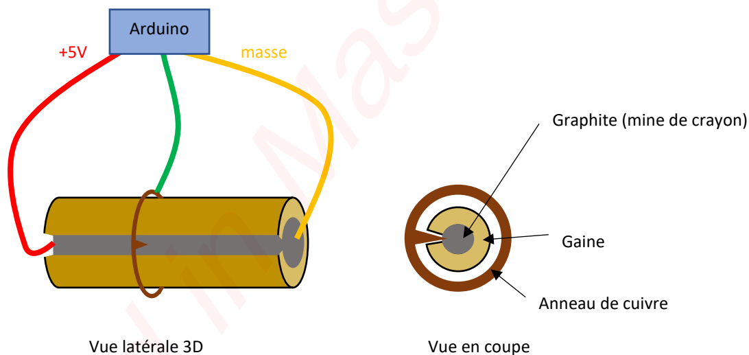
Figure 25 - Schéma du potentiomètre low-tech et du montage Arduino
