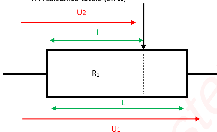
Figure 20 - Schéma de fonctionnement d'un potentiomètre
